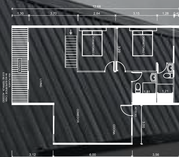
PRIMER PISO
