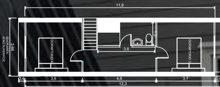
SEGUNDO PISO
